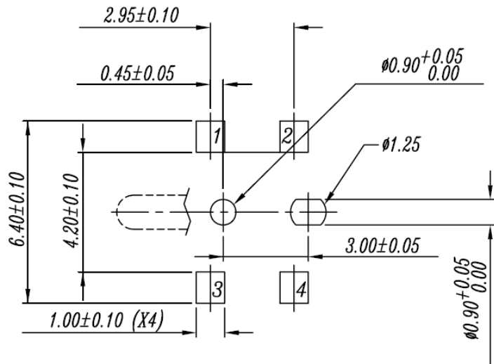
P.C.B LAYOUT
